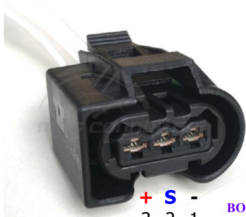
Fci/Delphi SICMA codice: M22122-K CONTROPARTE: M22127-K
