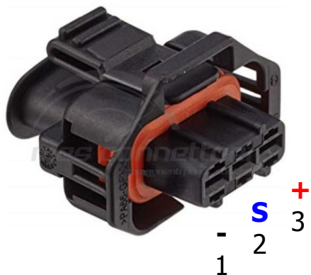
BOSCH COMPACT 3 vie p.f. codice: M3870-K (6901) CONTROPARTE: M4227-K (7224)
